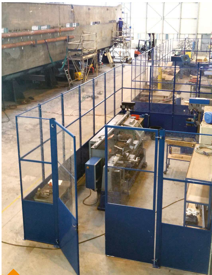
Intégration d'une cloison 5S pour créer un espace de travail sécurisé et protégé des courants d'air.
