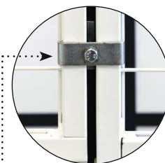
Assemblage des panneaux par pattes de fixation
