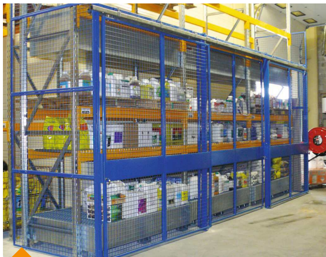
Cloison avec portes coulissantes pour limiter l'accès à des produits chimiques stockés dans des baies de rayonnage lourd, sur bacs de rétention.
