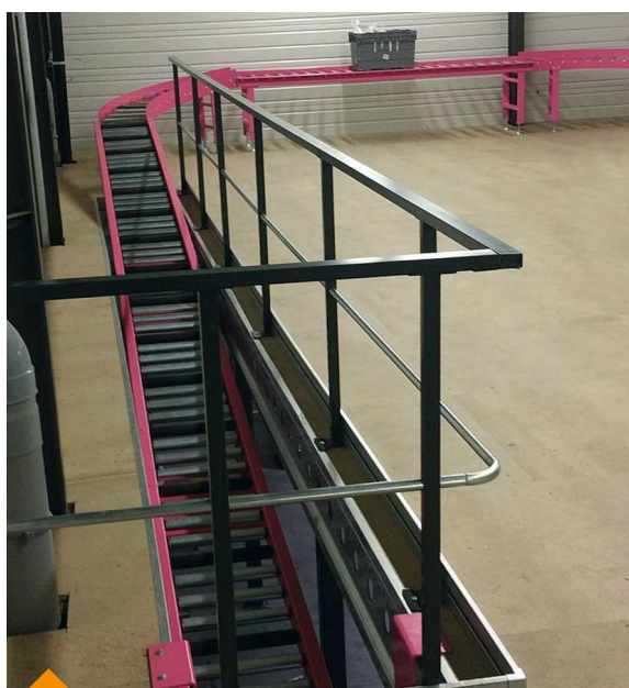
Plateforme avec intégration de convoyeur.
