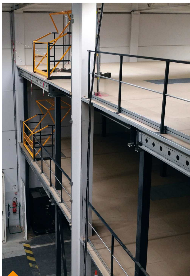
Plateforme 2 niveaux équipée de barrières écluse basculantes.
