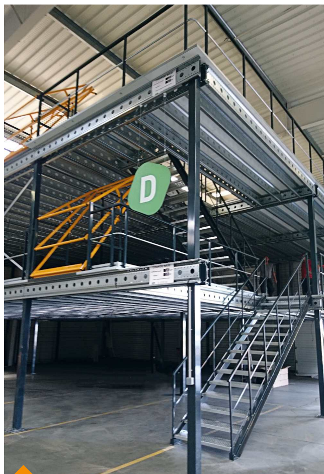
Plateforme avec escalier intégré et barrière écluse pliante.
