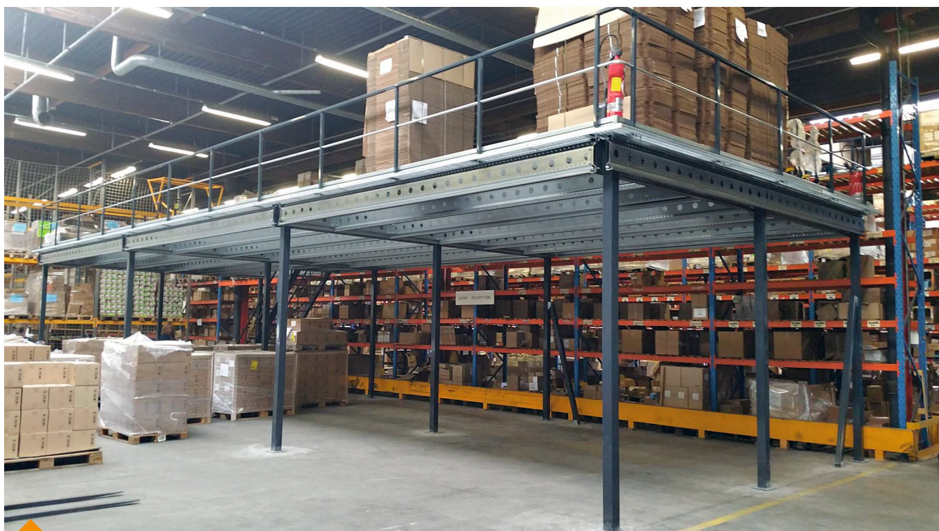
Plateforme autoportante : gagnez des mètres carrés supplémentaires.
