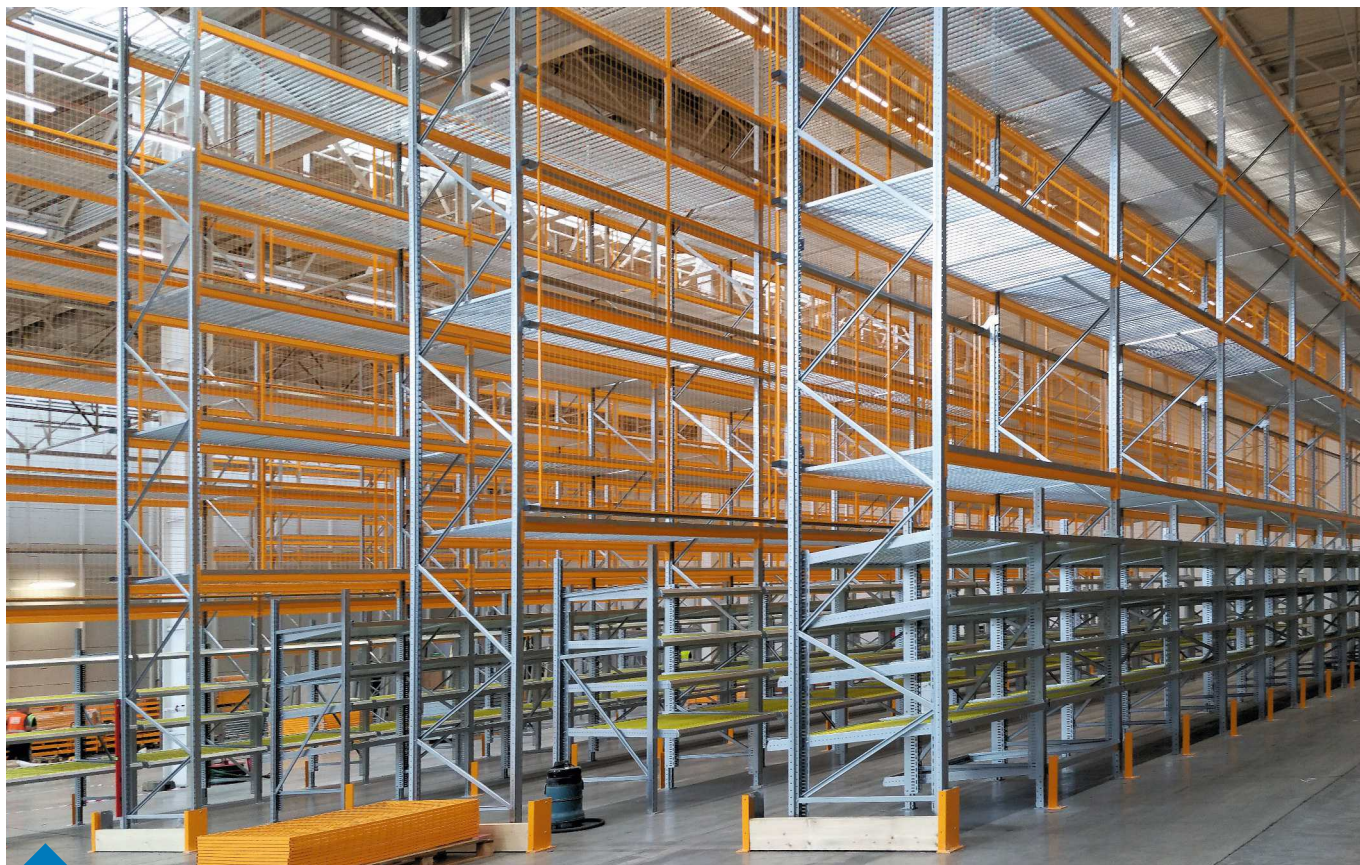
Installation de Propal 3 avec des nappes dynamiques aux niveaux inférieurs, pour le picking.
