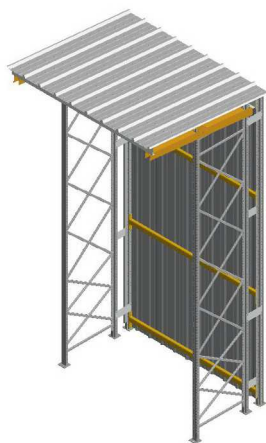
BAIE AVEC AUVENT ET BARDAGE ARRIÈRE
