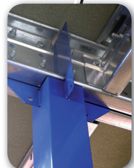
Encastrement tête de poteau.
