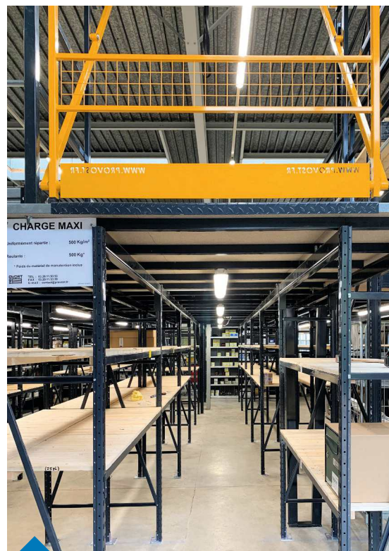
Le plancher de la plateforme repose sur les rayonnages Prorack+.
