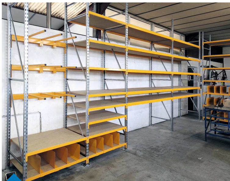
Meuble Prorack+ monté dans un atelier d'assemblage de vélos de course.
