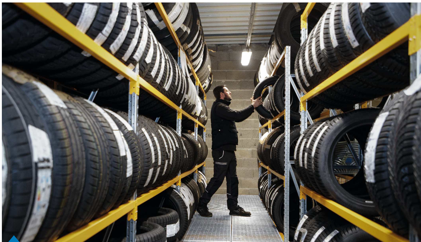
Plateforme avec allée de circulation en caillebotis sur des rayonnages Prorack+ pour le stockage de pneus en grande hauteur.
