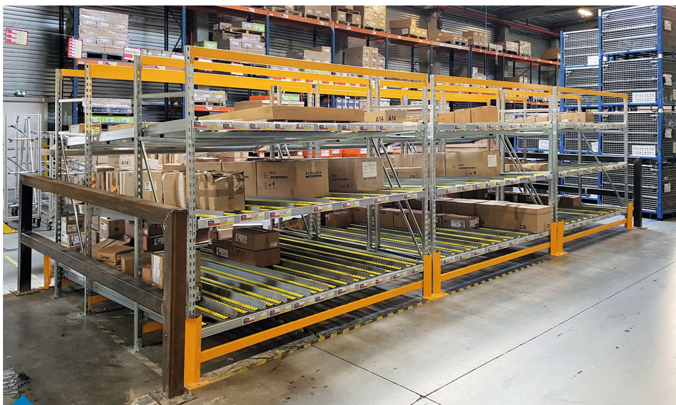
Prorack+ équipé de cadres dynamiques. Vue du côté du chargement à l'arrière du meuble. Les colis descendent de manière gravitaire jusqu'à la zone de prélèvement à l'avant.
