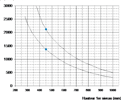
Charge (daN) CAPACITÉ PAR PAIRE DE MONTANTS
